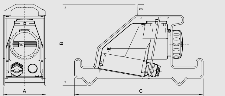
857./16-... соединительная муфта
